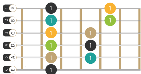
Reine Prime (0) / Reine Oktave (12)
